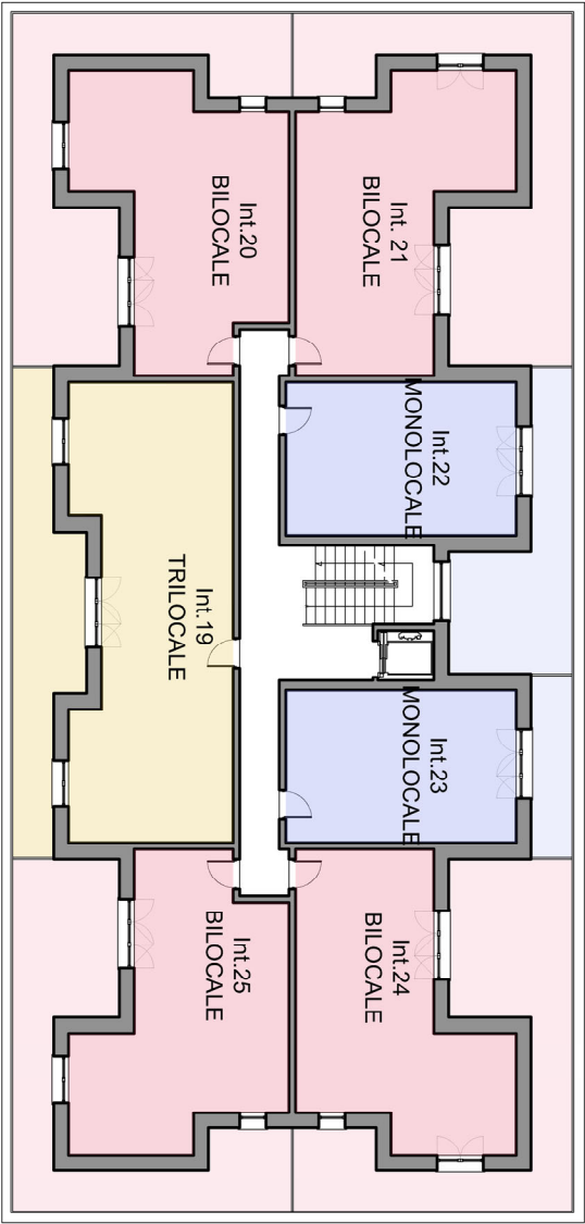
PIANTA PIANO TERZO
