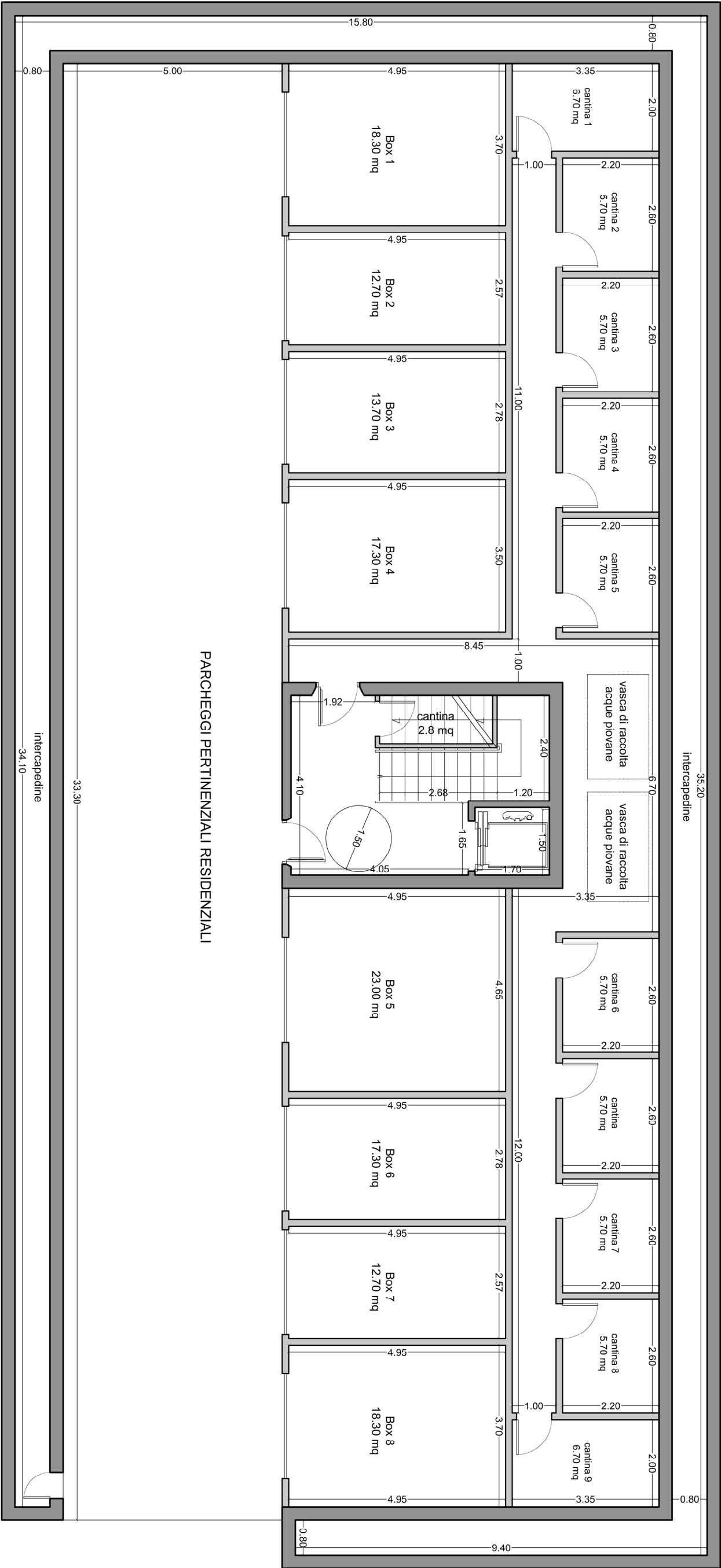
EDIFICIO A - PIANTA PIANO GARAGE
